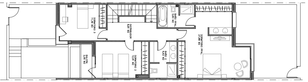
PLANTA PRIMERA
