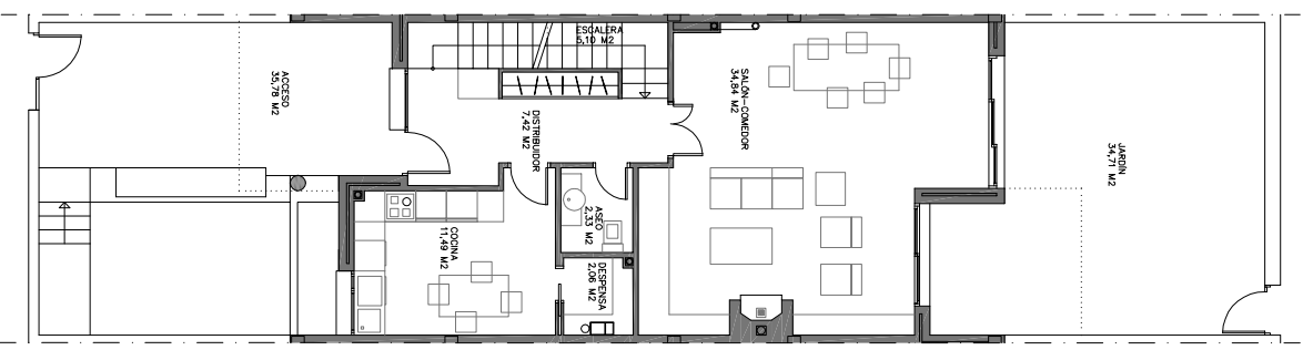
PLANTA BAJA
